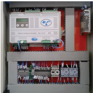
Quadro elétrico
